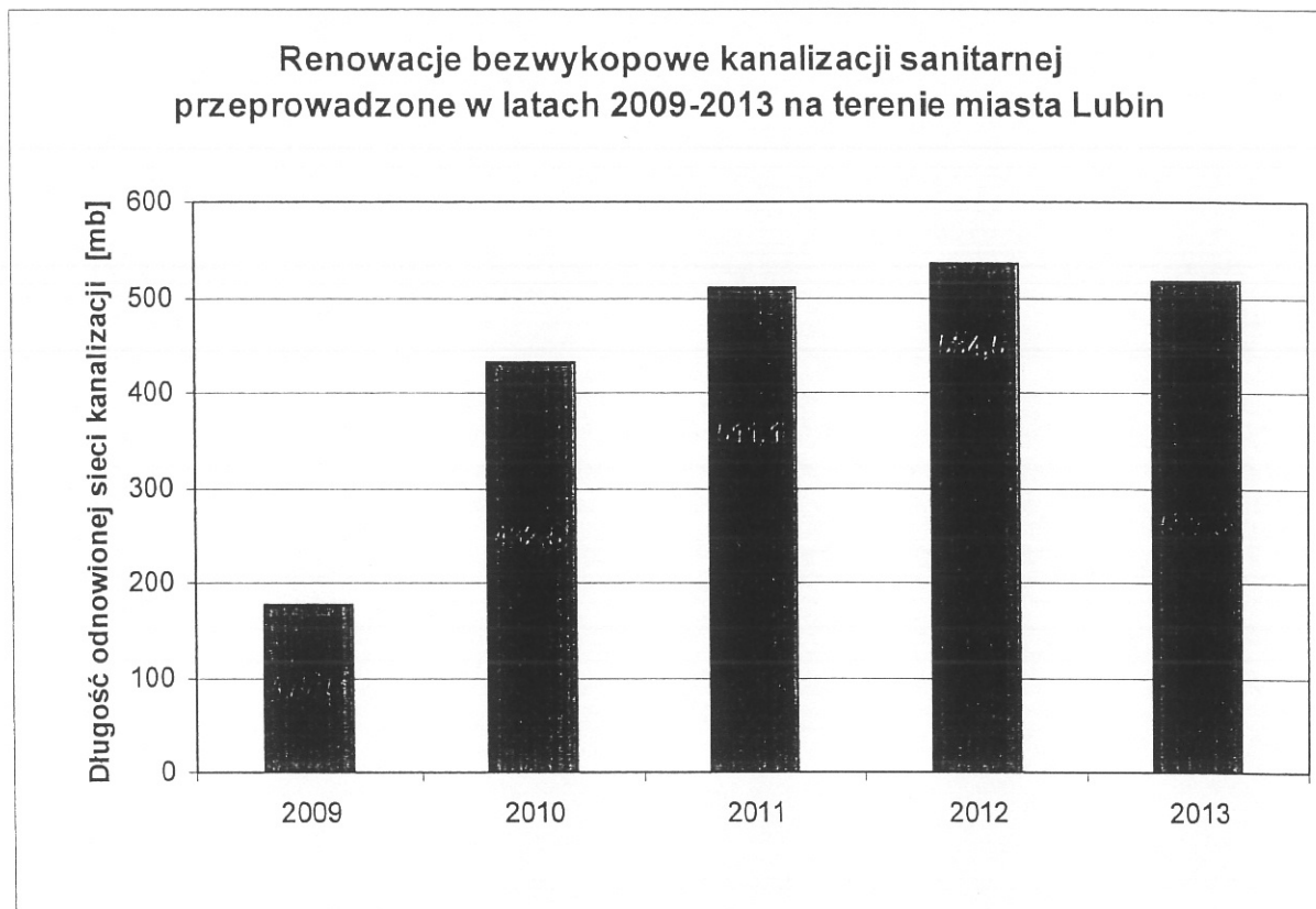
Wykres 3. Renowacje bezwykopowe sieci kanalizacji sanitarnej w latach 2009-2013 na terenie miasta Lubin.
